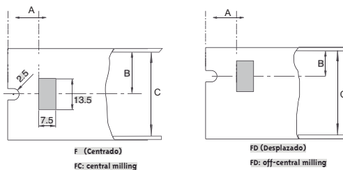
Dimensiones para mecanizado (mm)
