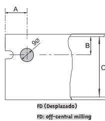
Dimensiones para mecanizado (mm)
