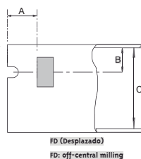
Dimensiones para mecanizado (mm)
