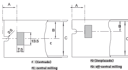
Dimensiones para mecanizado (mm)
