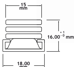
LA103-10-201 Compás limitador de fricción
