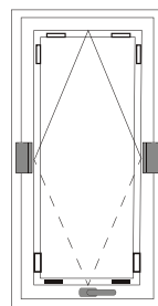
Pivotante
