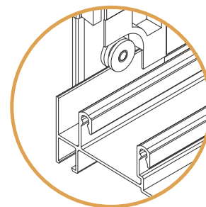
Mosquitera sobre guía inferior de ventana corredera
