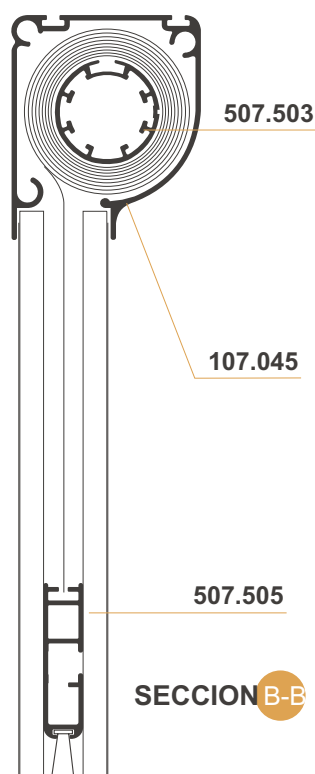
Guía Mosquitera Cepillo Convencional
