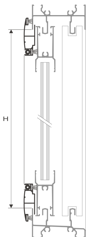
SECCION B-B
