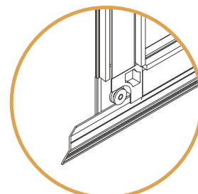
Mosquitera sobre carril adicional
