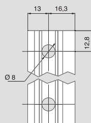
mecanizado en pletina falleba. mechanized of vertical rod.
