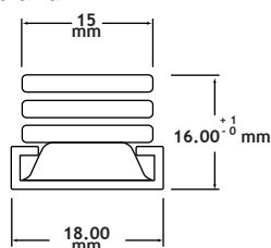
LA103-10-201 Compás limitador de fricción
